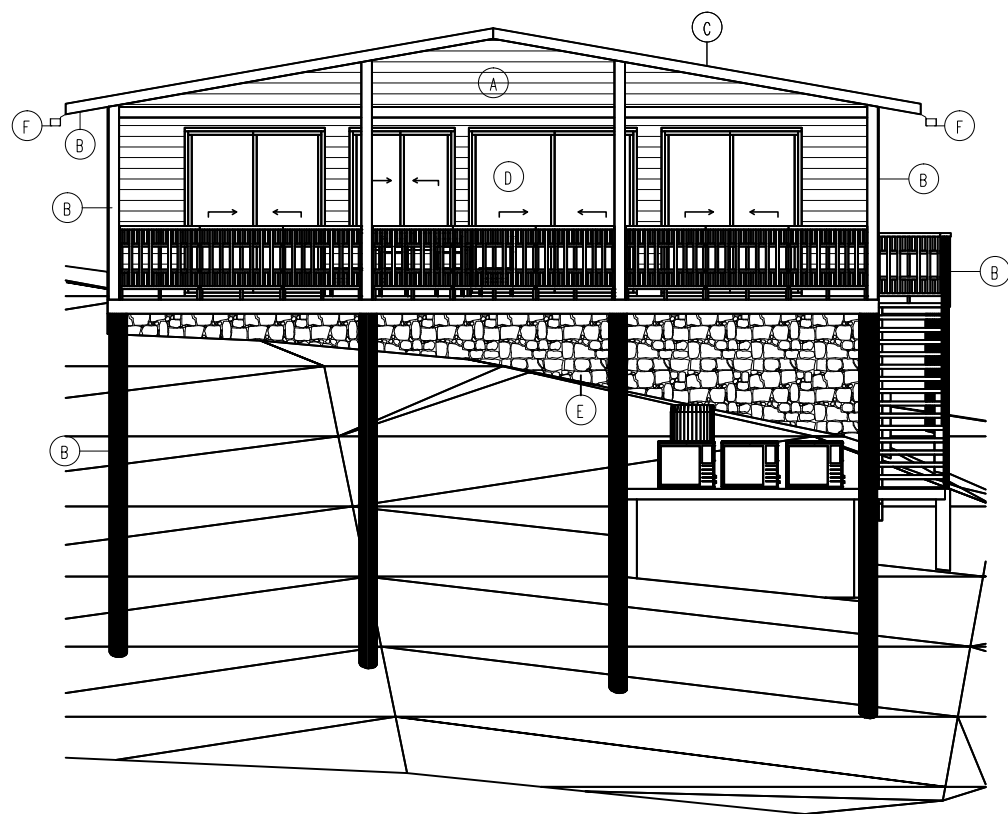
POHLED VÝCHODNÍ
