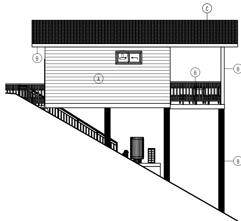
POHLED JIŽNÍ
