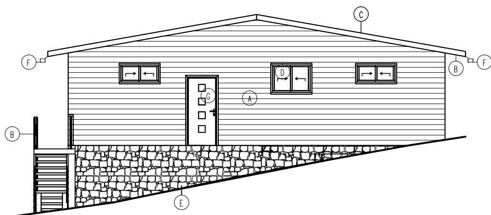
POHLED ZÁPADNÍ
